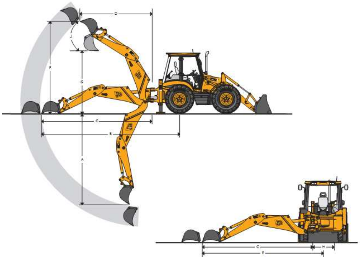
DIMENSIONES DE LA RETROEXCAVADORA
